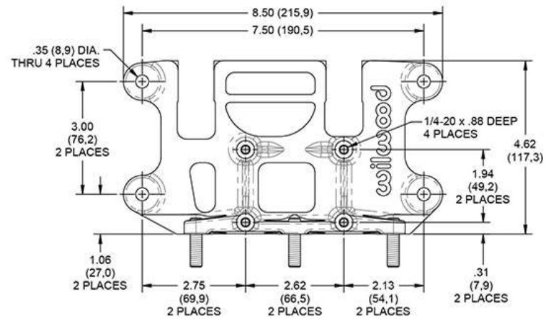
VIEW A-A
